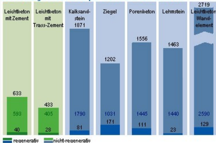
Primärenergiebedarf in MJ pro Kubikmeter Wandbaustoff
