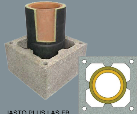
JASTO PLUS LAS FB Raumluftunabhängiger Betrieb für Festbrennstoffe. Die Frischluftzufuhr erfolgt über die Kanäle in den Ecken des Mantelsteins.
