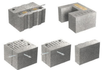
Das Jasto Quadro Lang System ist mit allen anderen Jasto Produkten kompatibel, beispielsweise mit dem Jasto Plan Therm (oben links), dem Jasto Säulenstein (oben rechts) und dem Jasto System-Laibungspaket (unten). Fotos: Jasto Baustoffwerke, Ochtendung
