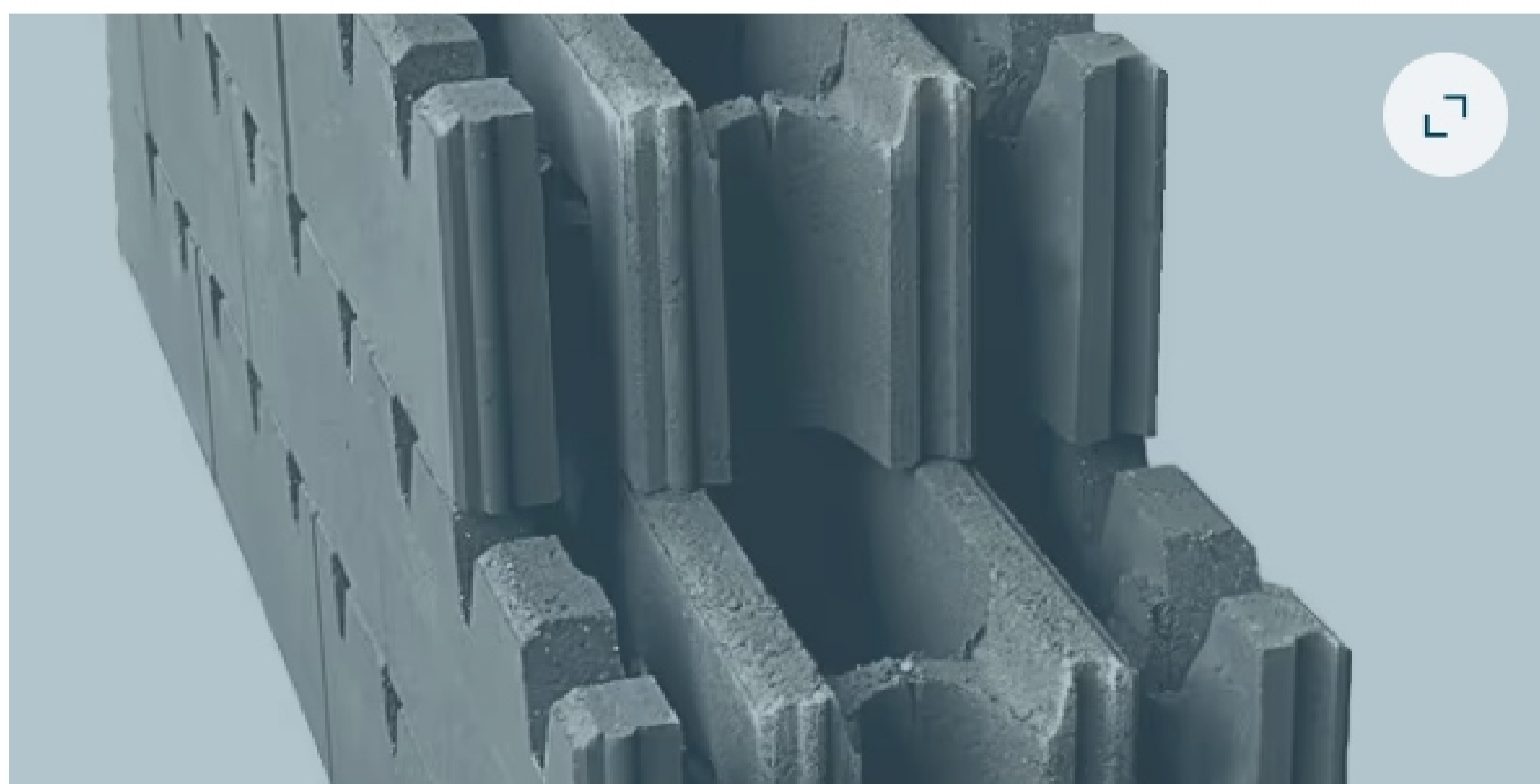
Die drei Kammern machen es möglich: Das „Green Wall-Kombi“-Mauersystem lässt sich außen ein- oder zweiseitig begrünen und innen ausbetonieren. | Foto: Jasto Baustoffwerke
