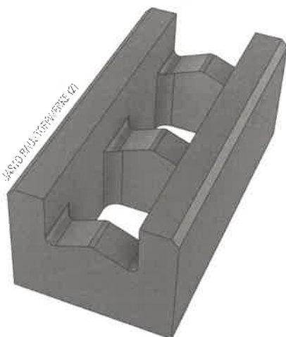
Der Grundstein der »Cavum-Mauer«. Ergänzt wird er zusätzlich durch einen langen und einen kurzen Endstein.
